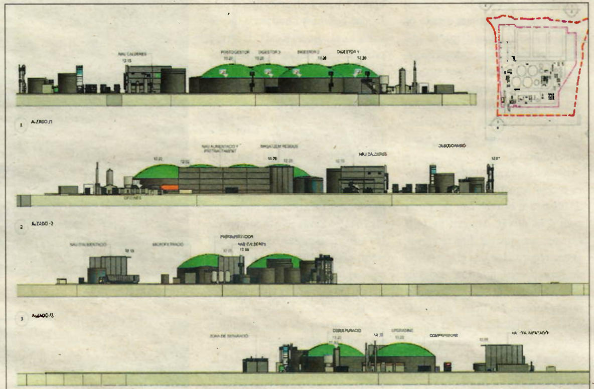
Alçats de la proposta de la planta de biometà que es projecta al costat del polígon industrial Catalunya Sud.
